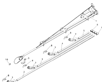
ETB-011667, 20 m - zewnętrzny wysięgnik, prawy
