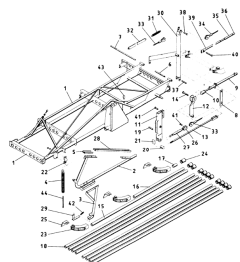
ETB-011663, 20 m - wewnętrzny wysięgnik, prawy
