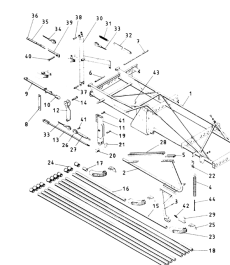
ETB-011662, 20 m - wewnętrzny wysięgnik, lewy
