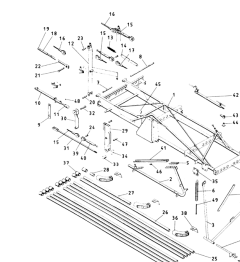
ETB-011674, 24 m - wewnętrzny wysięgnik w pełni hydr., lewy
