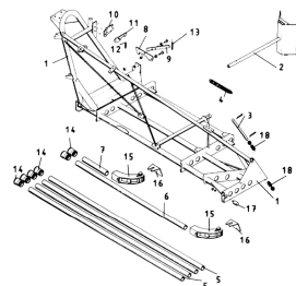
ETB-011664, 20 m - część środkowa wysięgnika, lewa
