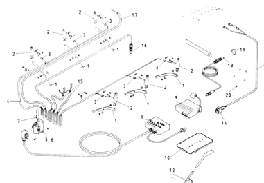
ETB-011661, Układ przełączający i sterujący
