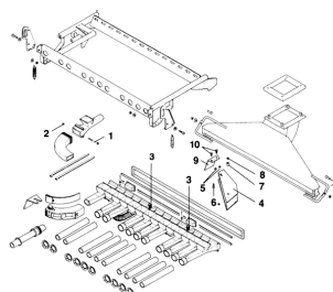
ETB-011659, Kanał powietrza i iniektory, prawa strona (2/2)
