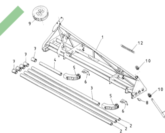
ETB-011678, 24 m - część wewnętrzna zewnętrznego wysięgnika w pełni hydr., lewa
