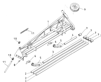
ETB-011679, 24 m - część wewnętrzna zewnętrznego wysięgnika w pełni hydr., prawa
