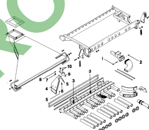
ETB-011657, Kanał powietrza i iniektory, lewa strona
