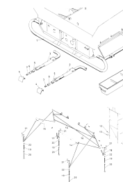
ETB-011686, Napęd Super Jet
