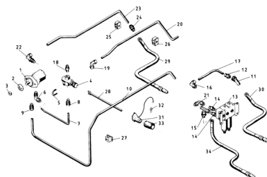
ETB-011655, Napęd hydrostatyczny (1/2)
