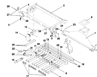
ETB-011658, Kanał powietrza i iniektory, prawa strona (1/2)
