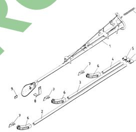
ETB-011681, 24 m - część zewnętrzna zewnętrznego wysięgnika w pełni hydr., prawa
