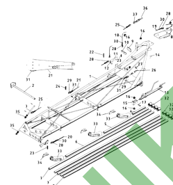
ETB-011677, 24 m - część środkowa wysięgnika w pełni hydr., prawa
