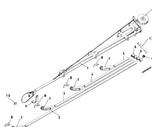
ETB-011673, 20 m - zewnętrzny wysięgnik w pełni hydr., prawy
