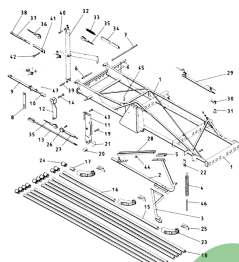
ETB-011668, 20 m - wewnętrzny wysięgnik w pełni hydr., lewy
