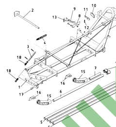
ETB-011665, 20 m - część środkowa wysięgnika, prawa
