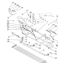
ETB-011670, 20 m - część środkowa wysięgnika w pełni hydr., lewa
