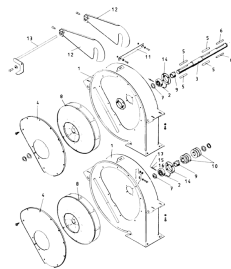
ETB-011652, Dmuchawa, redukcja powietrza kompl.
