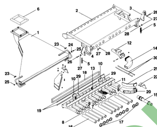
ETB-011656, Napęd hydrostatyczny (2/2)
