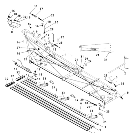
ETB-011676, 24 m - część środkowa wysięgnika w pełni hydr., lewa
