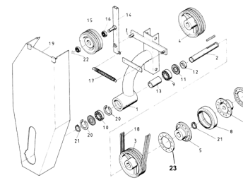
ETB-011685, Napęd Super Jet
