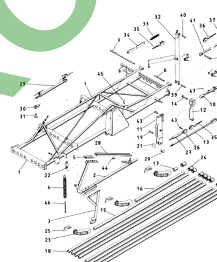
ETB-011669, 20 m - wewnętrzny wysięgnik w pełni hydr., prawy
