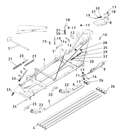
ETB-011671, 20 m - część środkowa wysięgnika w pełni hydr.
