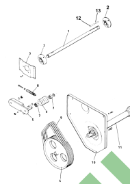
ETB-011653, Napęd dmuchawy
