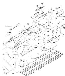
ETB-011675, 24 m - wewnętrzny wysięgnik w pełni hydr., prawy
